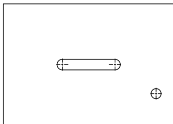
К-4 (Верхняя панель 324x230x16) - 1 шт
