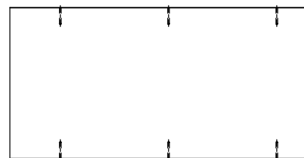
К-3 (Задняя панель 968x328x16) - 1 шт
