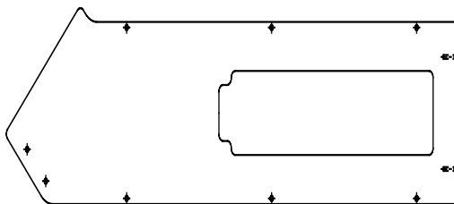
К-2 (Боковина 1096x260x16) - 2 шт
